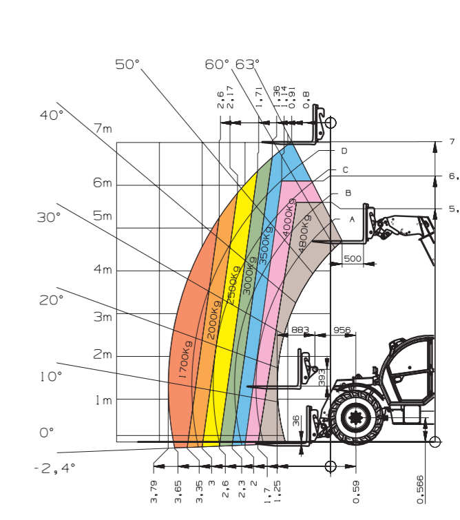
KT507 Esquema de capacidad de carga (con LSP 500 mm)
