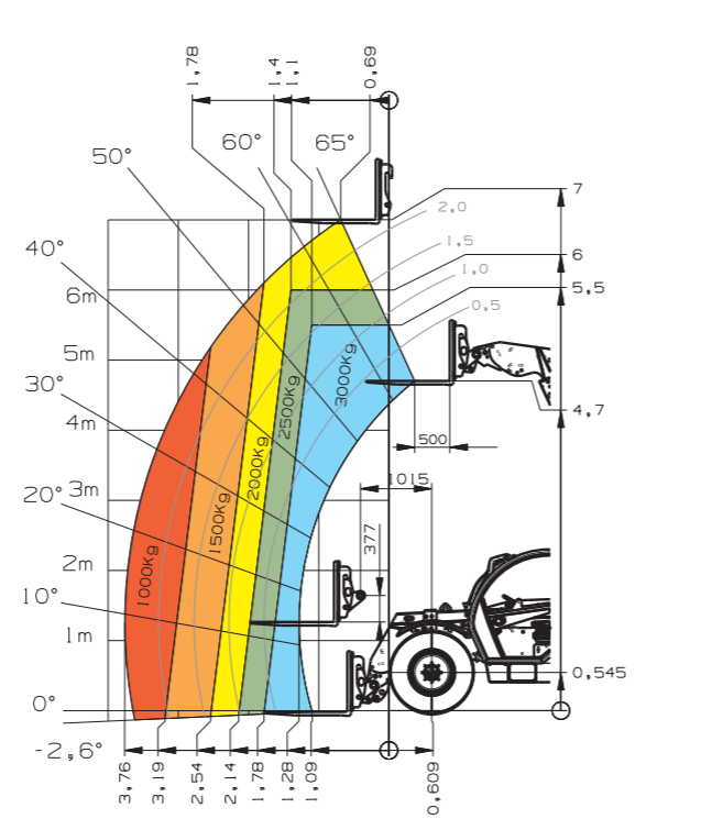
KT307 Esquema de capacidad de carga (con LSP 500 mm)
