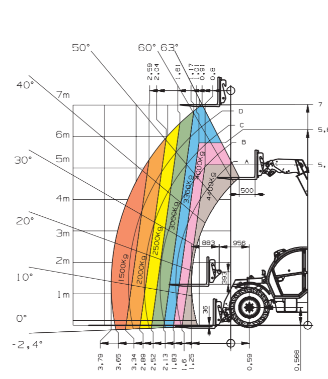
KT447 Esquema de capacidad de carga (con LSP 500 mm)
