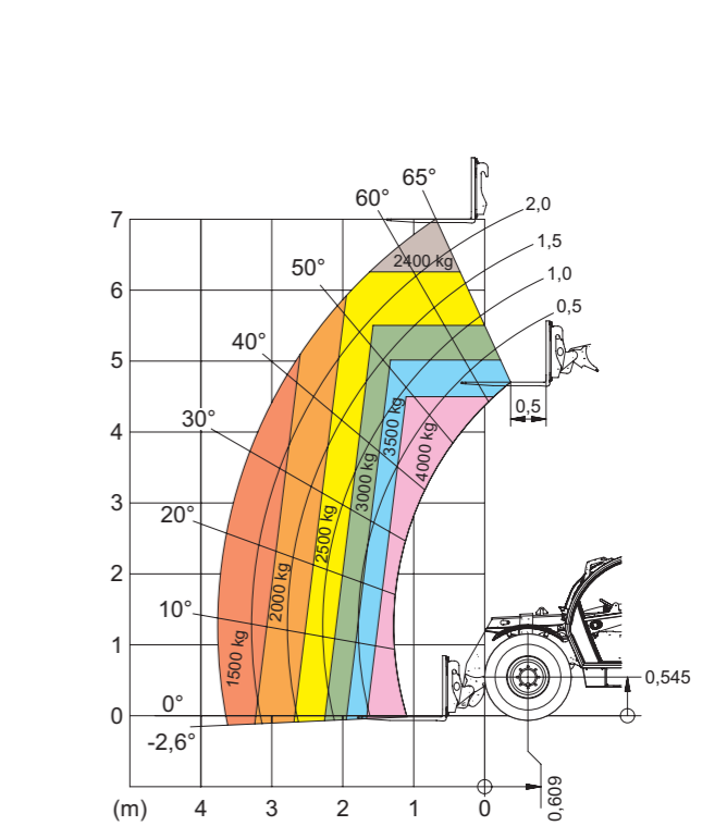
KT407 Esquema de capacidad de carga (con LSP 500 mm)
